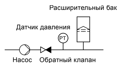
Рис. 31 Положение обратного клапана и датчика давления в системе с положительным давлением на входе
